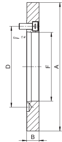
FLANSCH VORGEARBEITET SEMI-MACHINED ADAPTER PLATES
